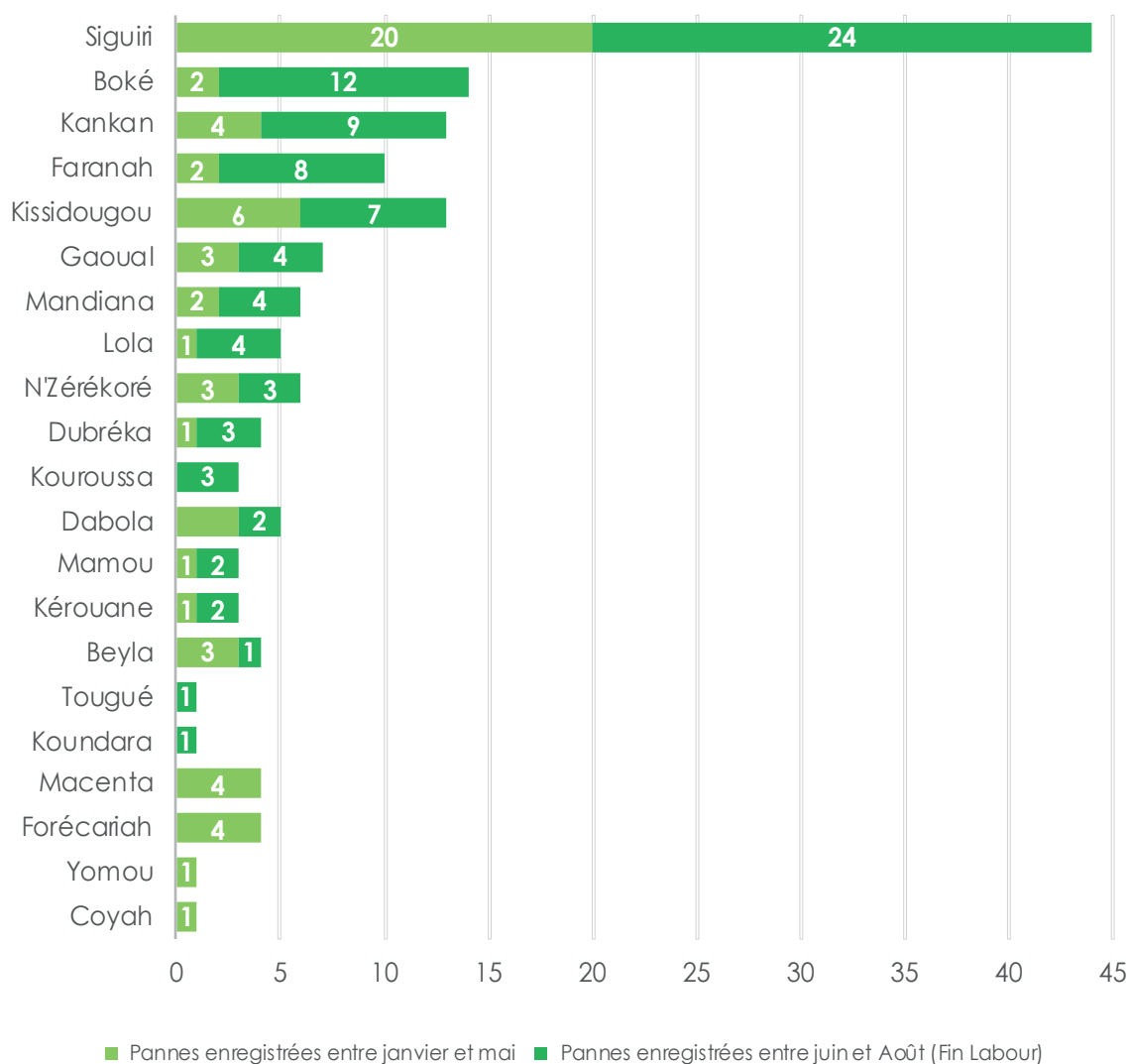
G23 : Suivi de pannes remontées par CPA
